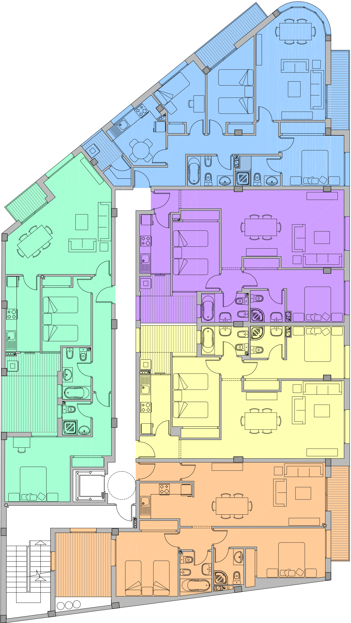
PLANTA PISO 1°
