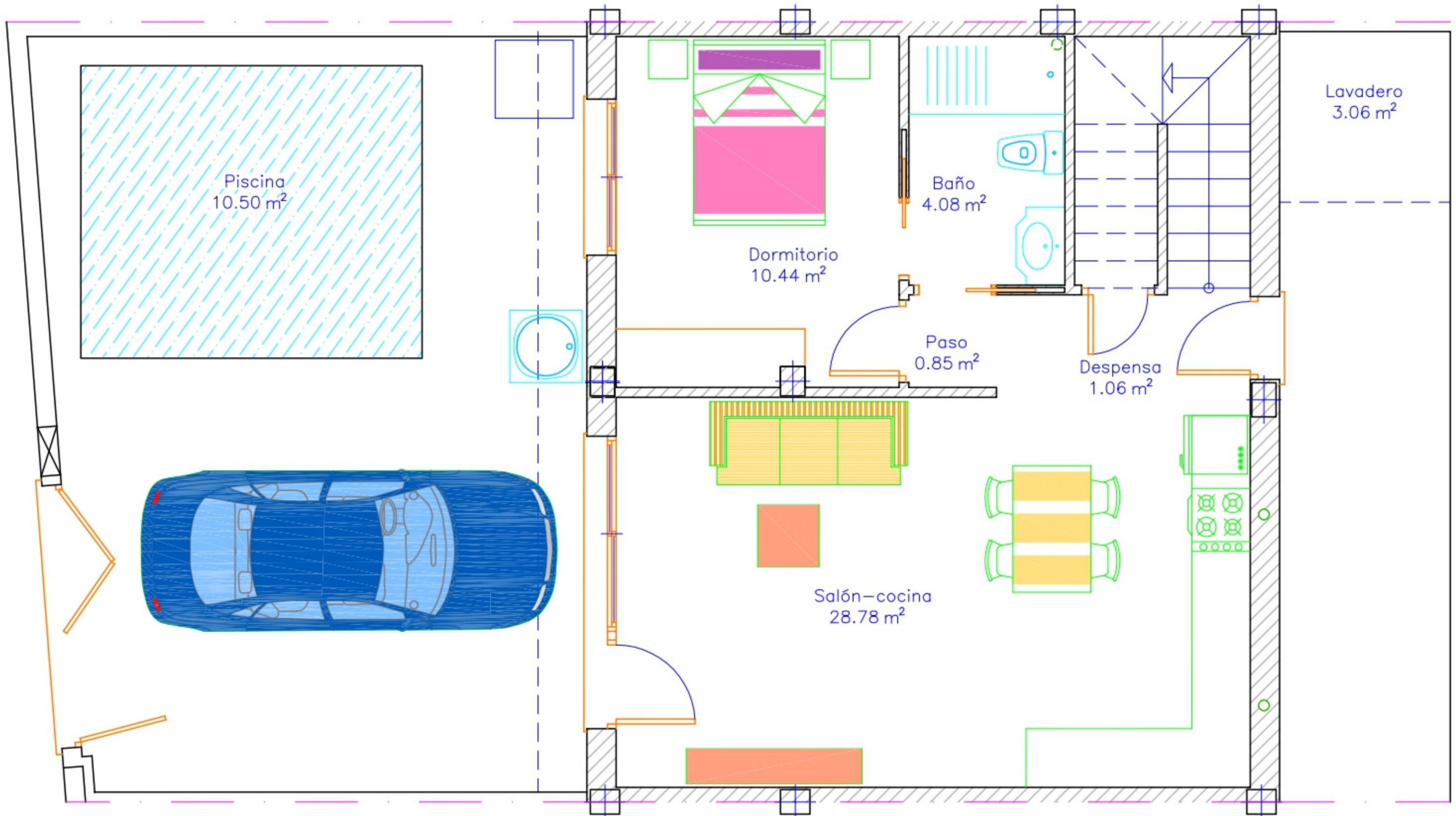
PLANTA 0, S.C.= 62.03M2
