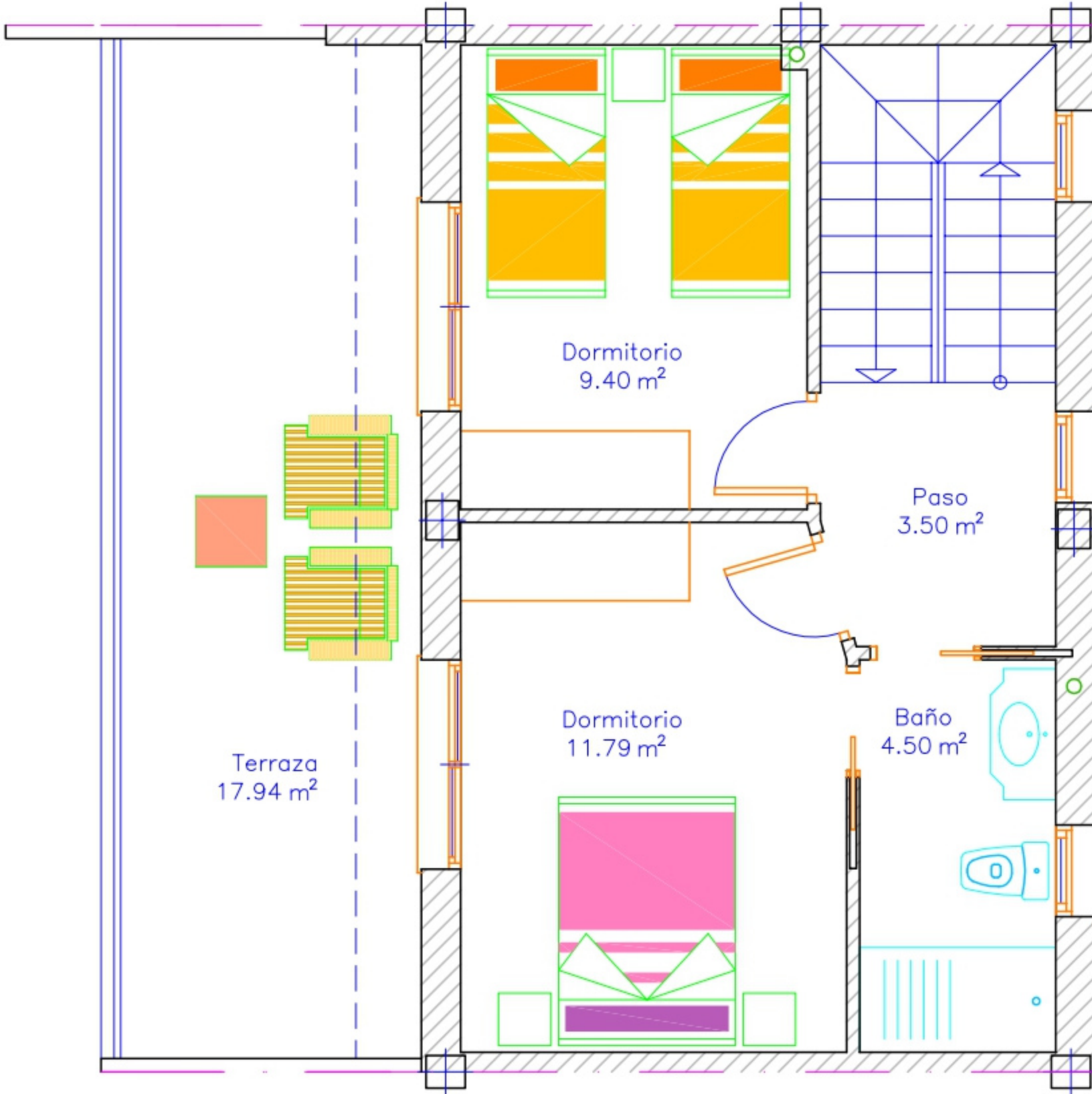
PLANTA 1, S.C.= 43.20 M2
