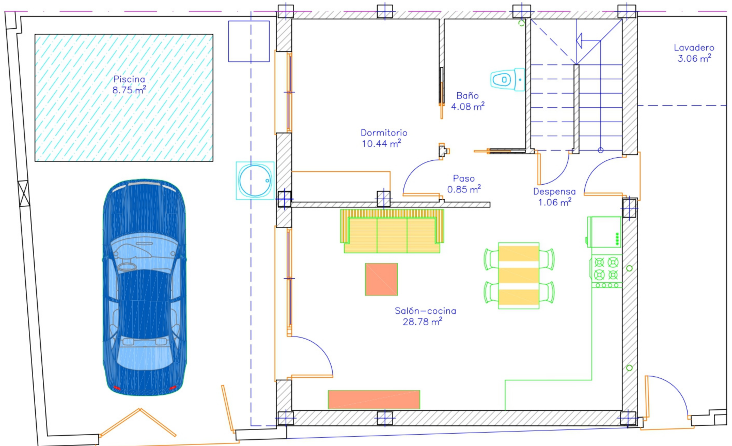
PLANTA 0, S.C.= 63.14M2
