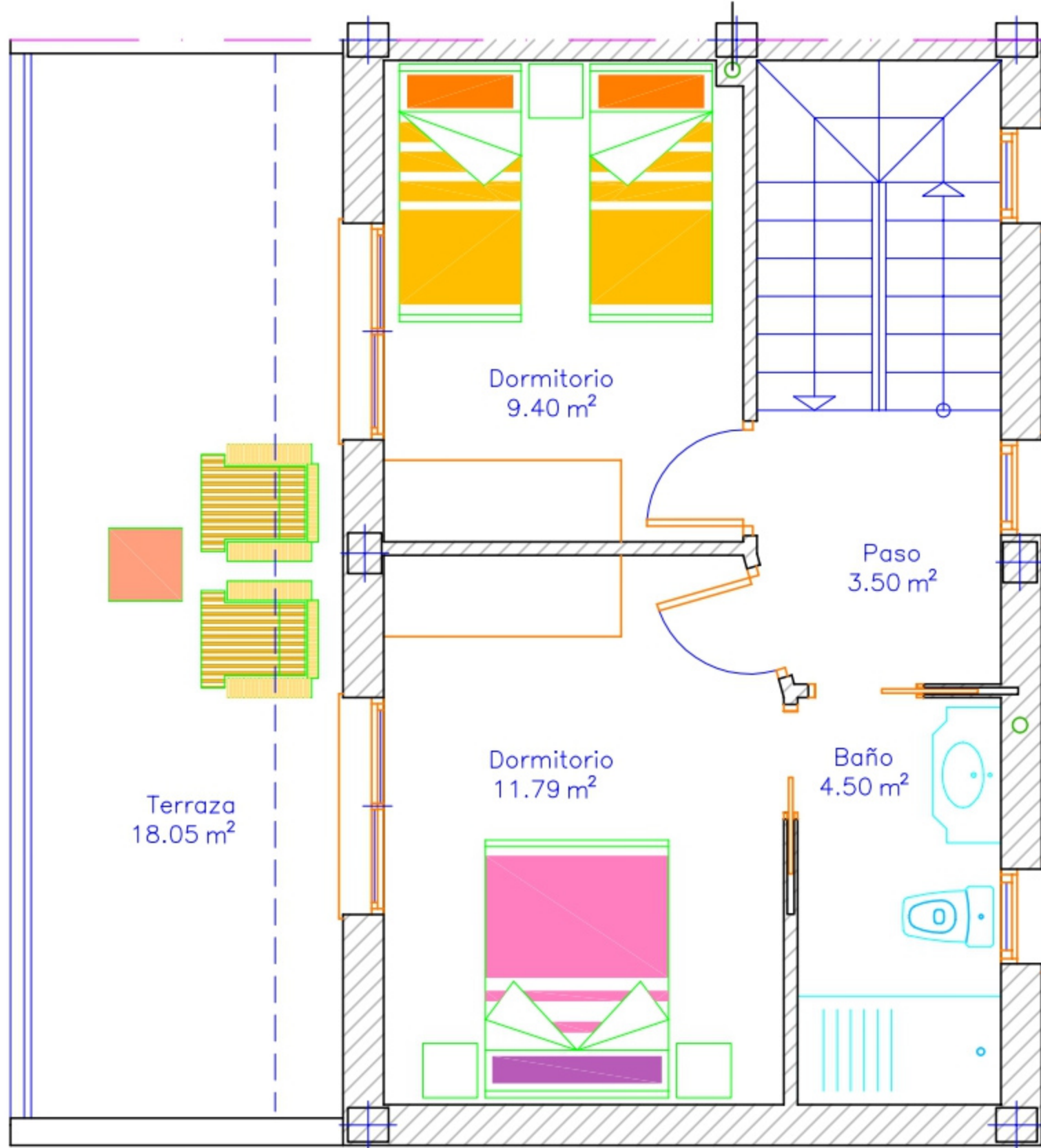
PLANTA 1, S.C.= 44.01M2
