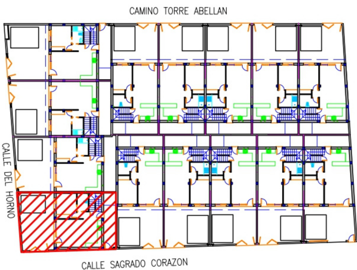
PLANTA 0, S.C.= 63.14M2
