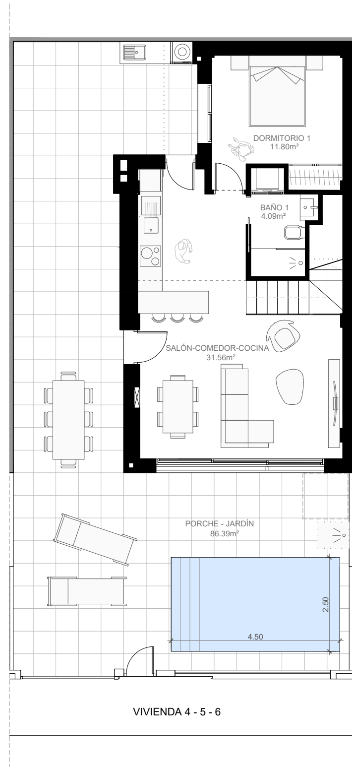
PLANTA BAJA
