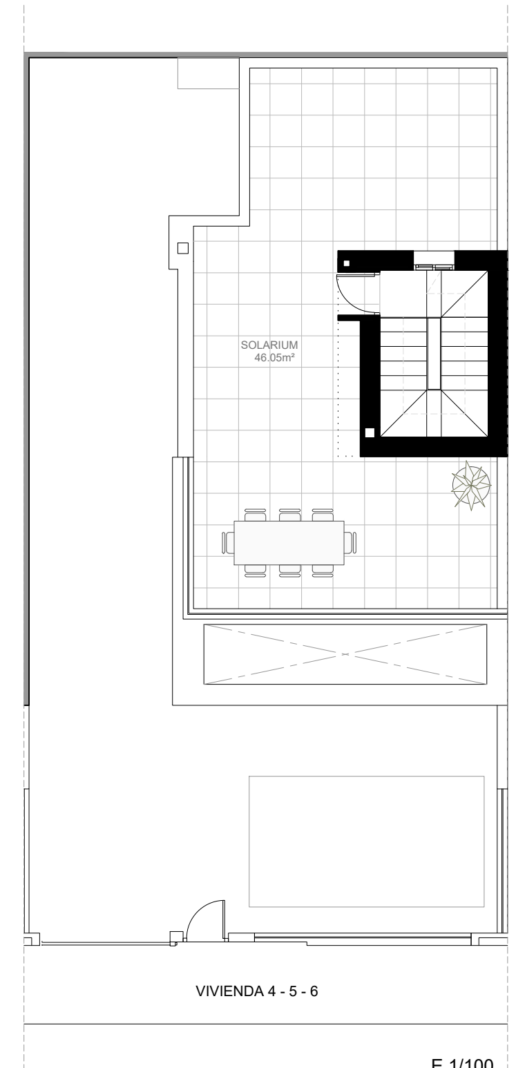
PLANTA SOLARIUM
