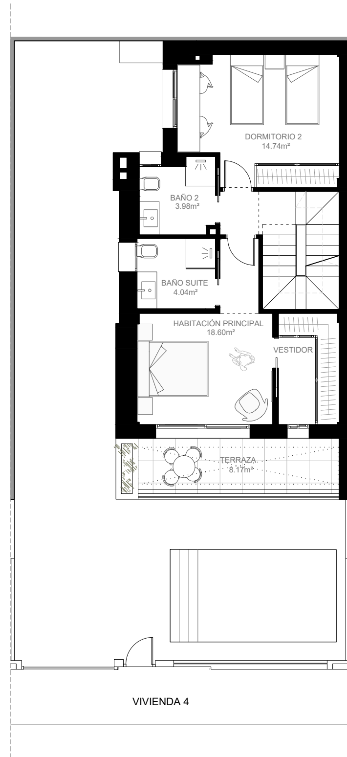
PLANTA PRIMERA
