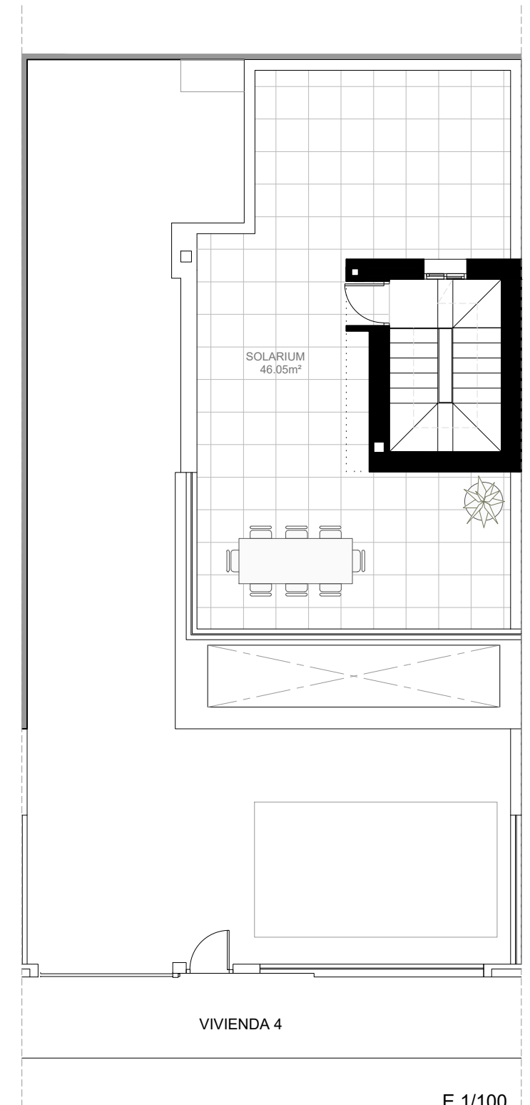
PLANTA SOLARIUM
