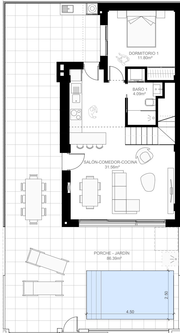
PLANTA BAJA
