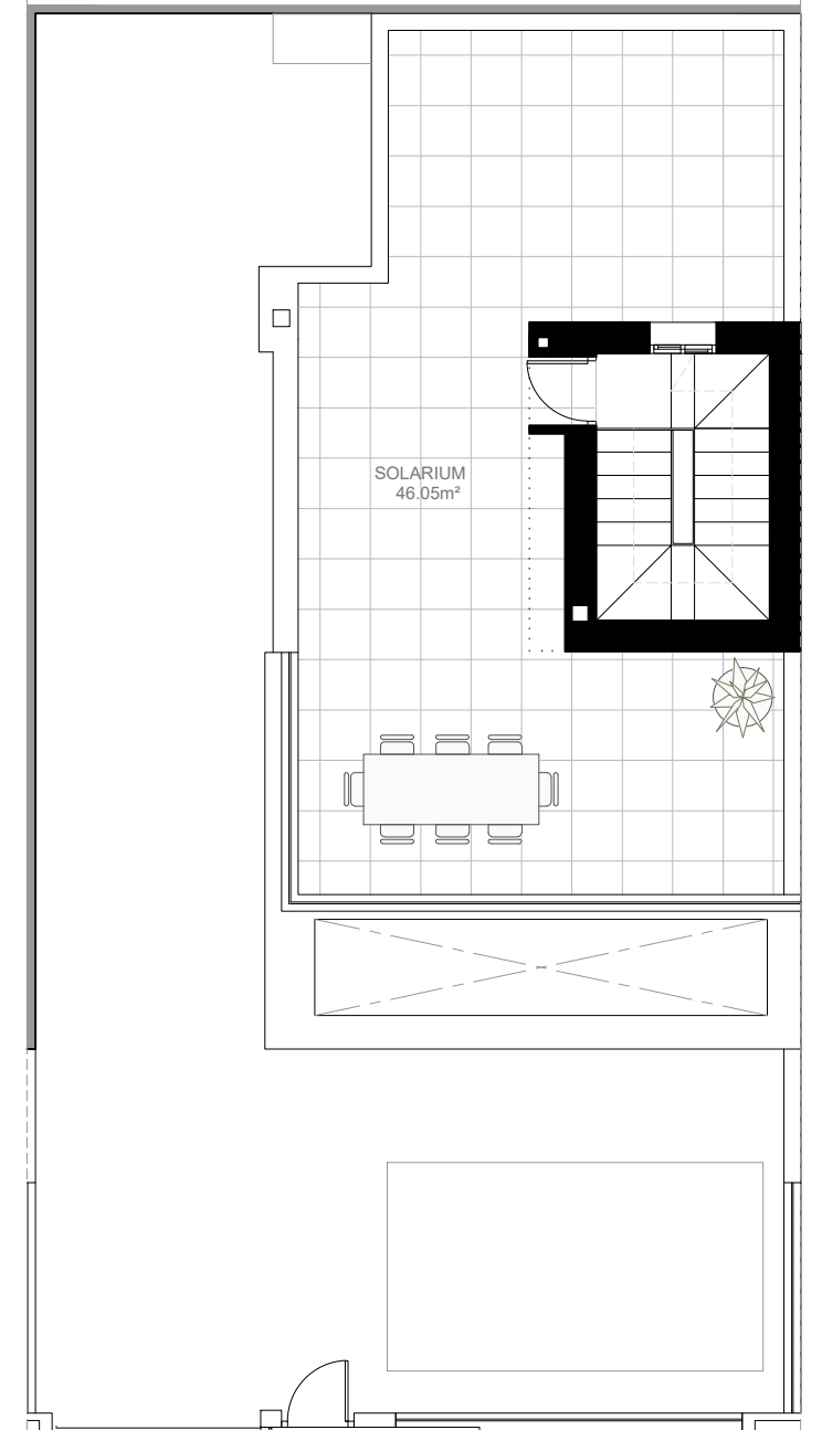
PLANTA SOLARIUM
