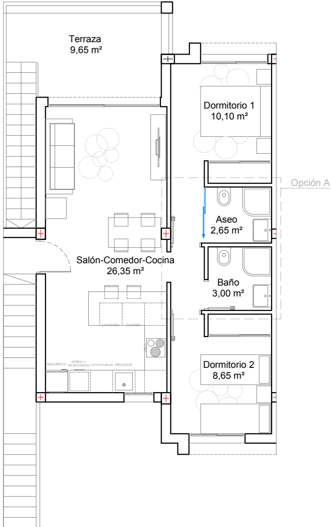
PLANTA ALTA | Superficie 60 m 2
