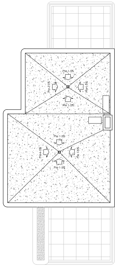
PLANTA CUBIERTA
