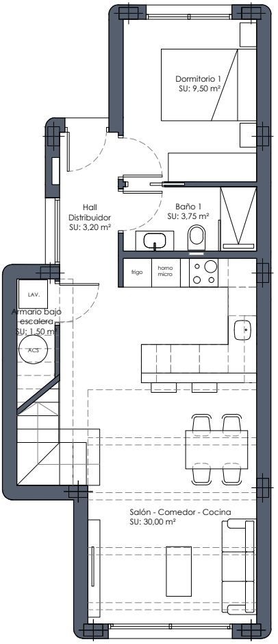
PLANTA BAJA
