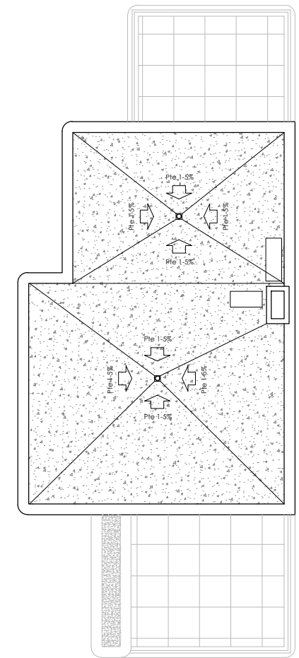
PLANTA CUBIERTA
