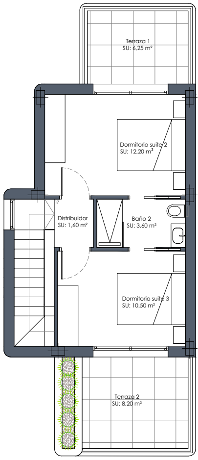
PLANTA PRIMERA
